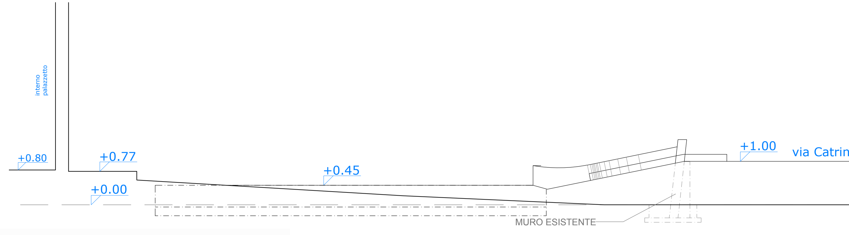
SEZIONE 1 _ SCALA 1:50
