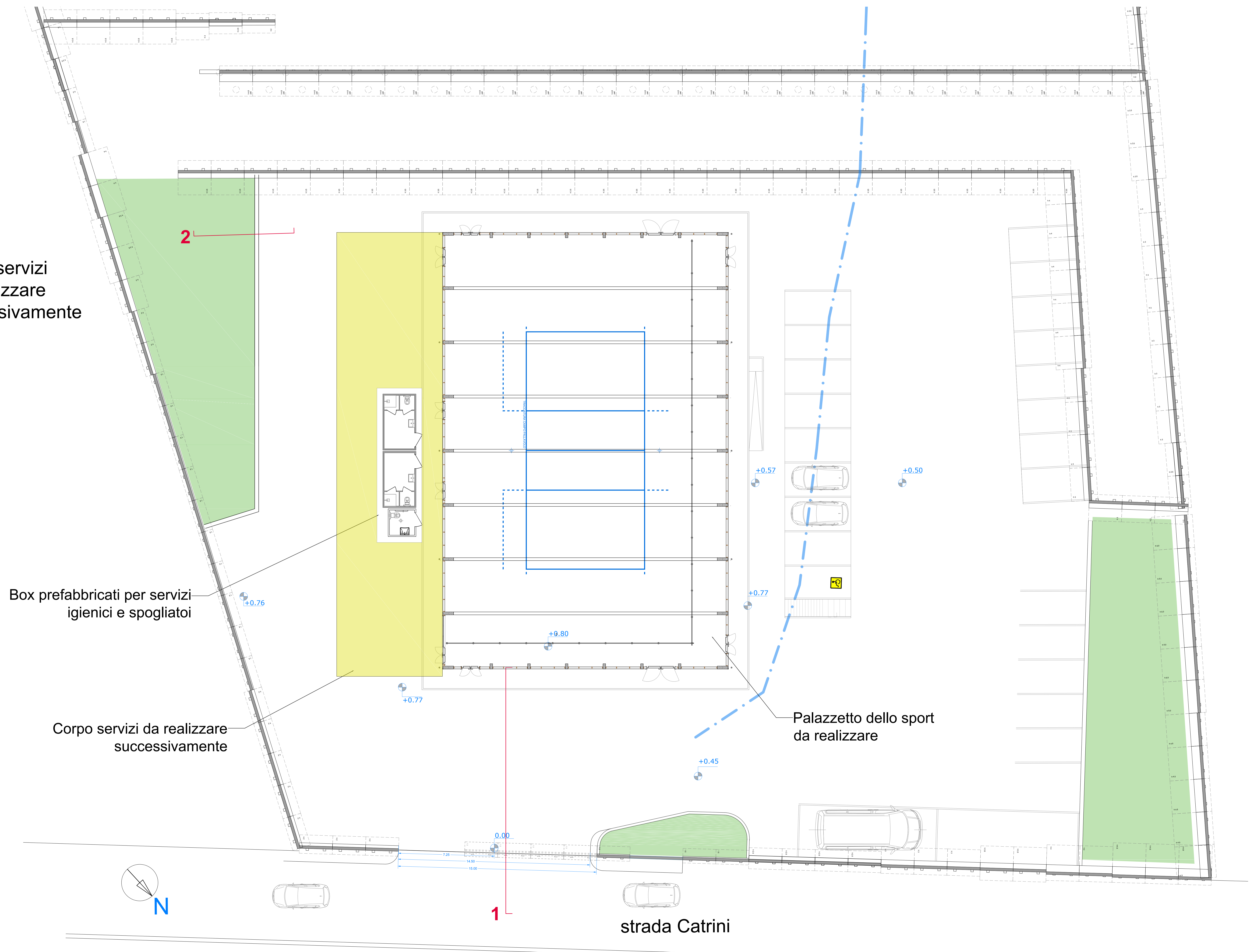
PLANIMETRIA _ SCALA 1:100
