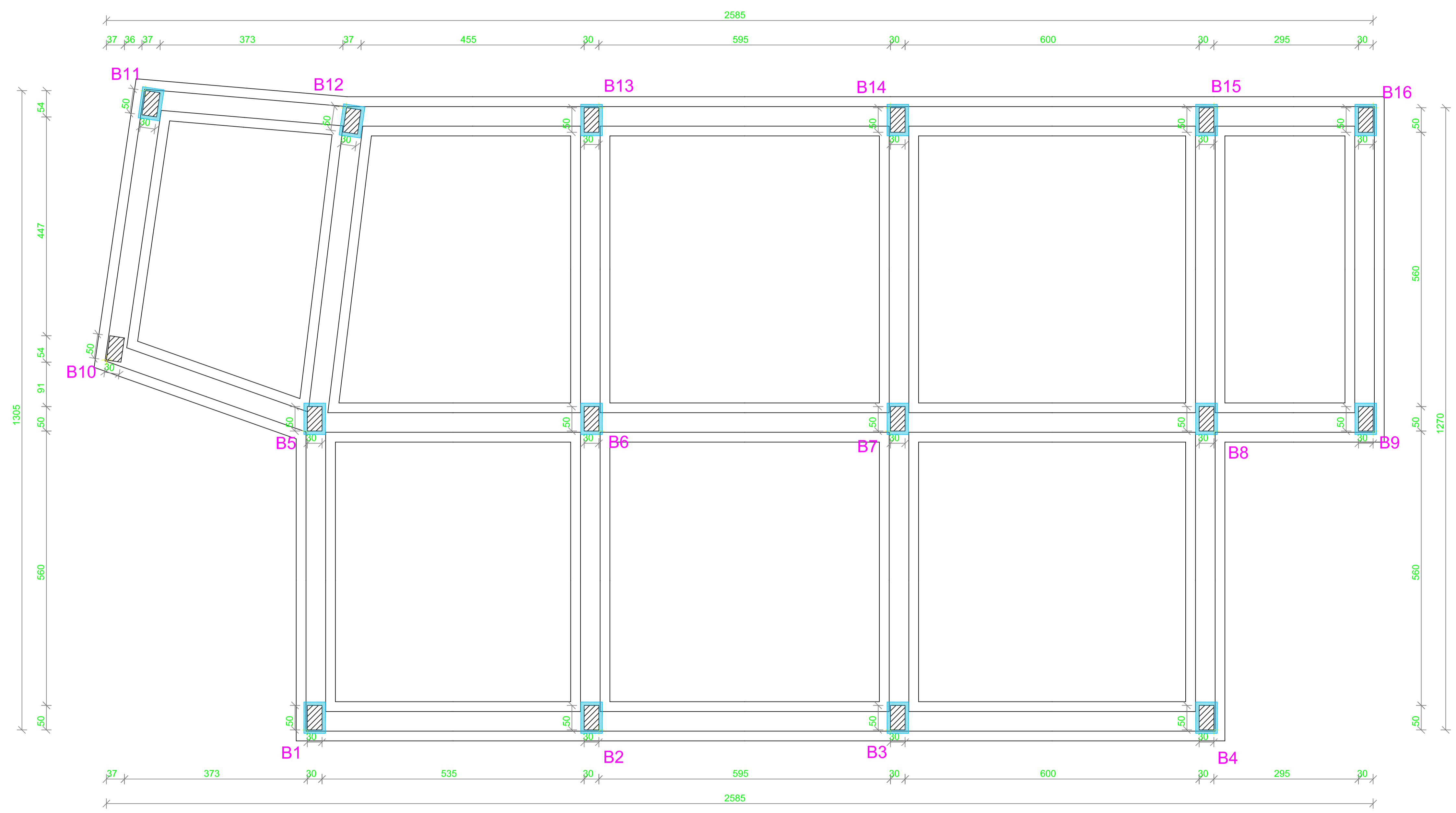
STRUTTURA "B" PIANTA IMPALCATO QUOTA m: 0.00
