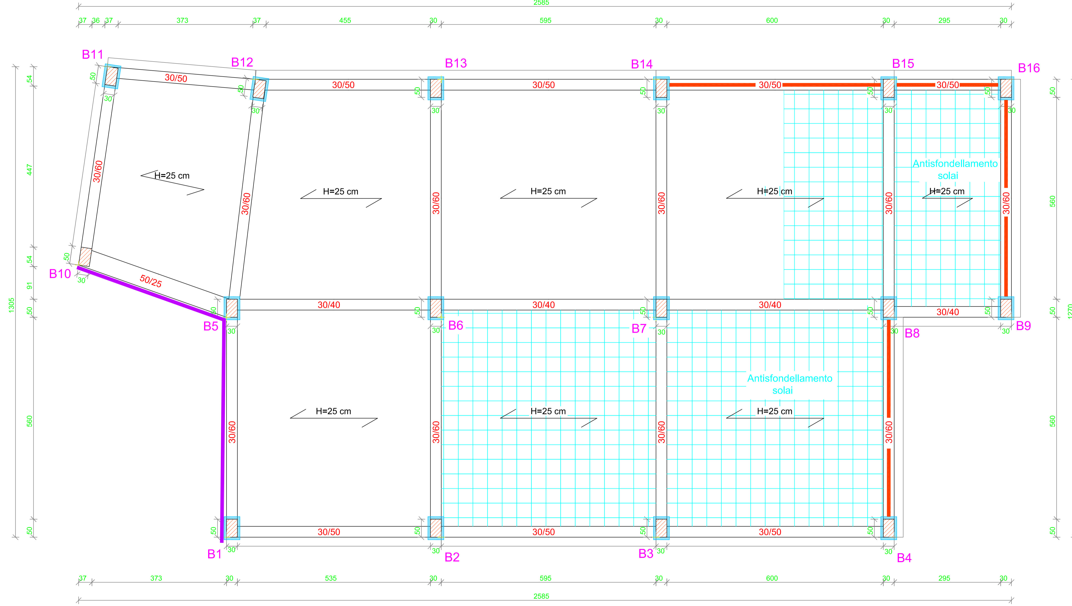
STRUTTURA "B" - PIANTA COPERTURA - IMPALCATO QUOTA m: 5.10
