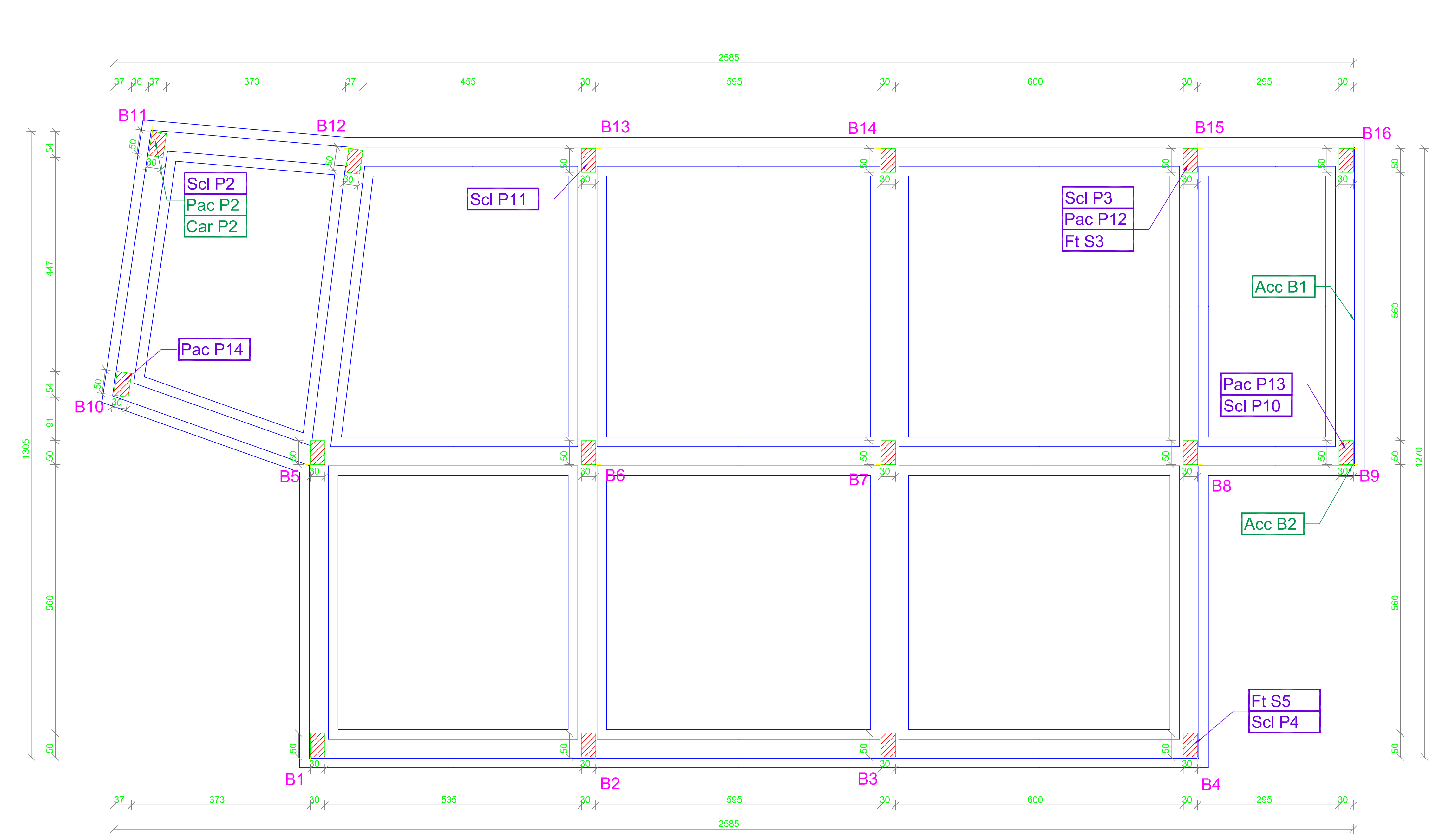
STRUTTURA "B" PIANTA IMPALCATO QUOTA m: 0.00
