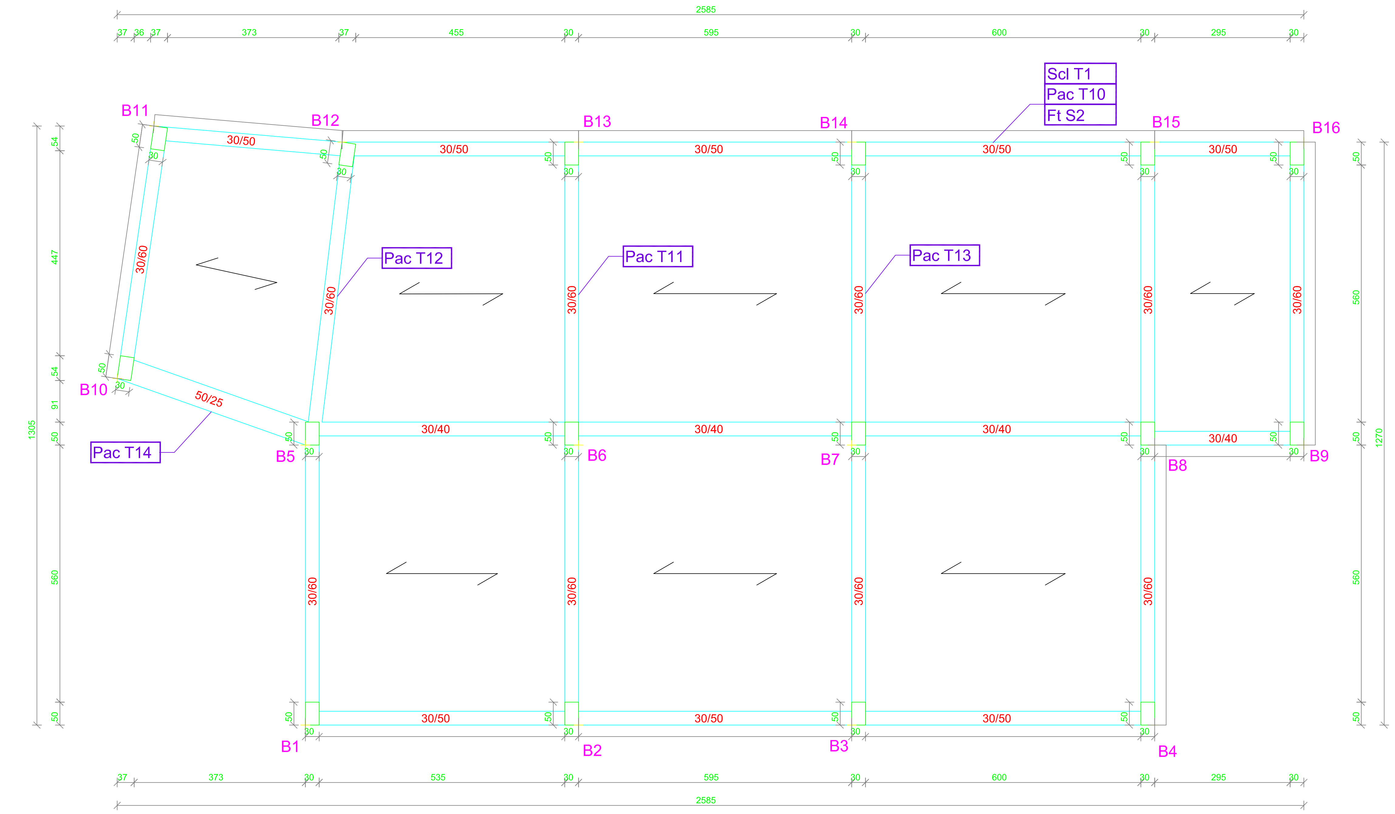
STRUTTURA "B" - PIANTA COPERTURA - IMPALCATO QUOTA m: 5.10
