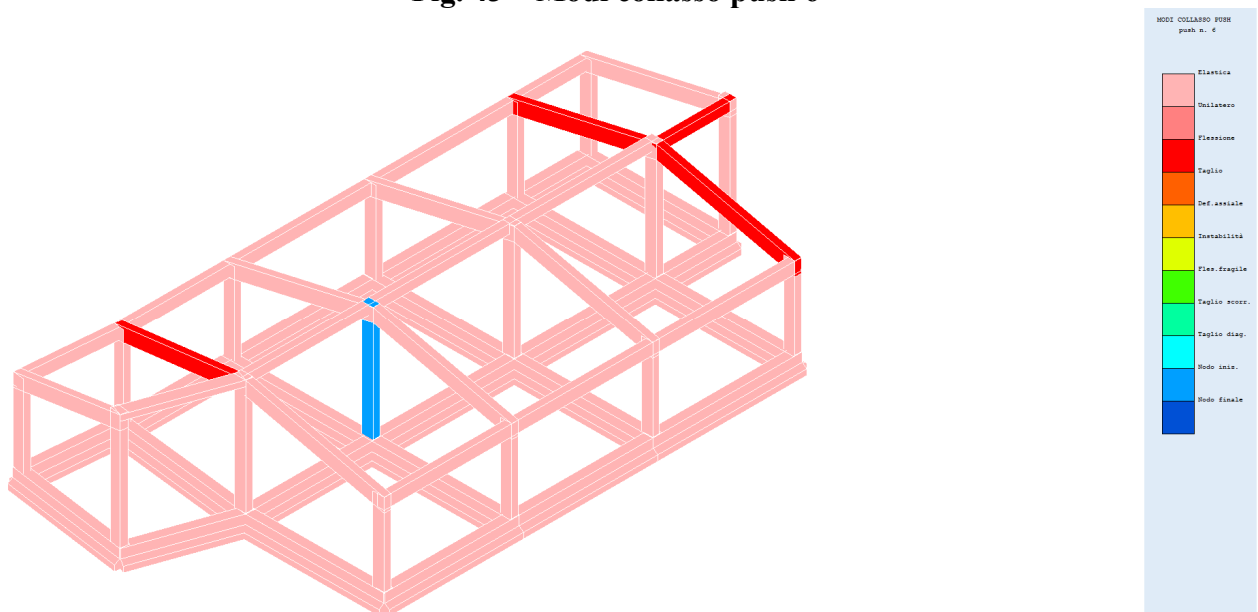
Fig. 43 – Modi collasso push 6
