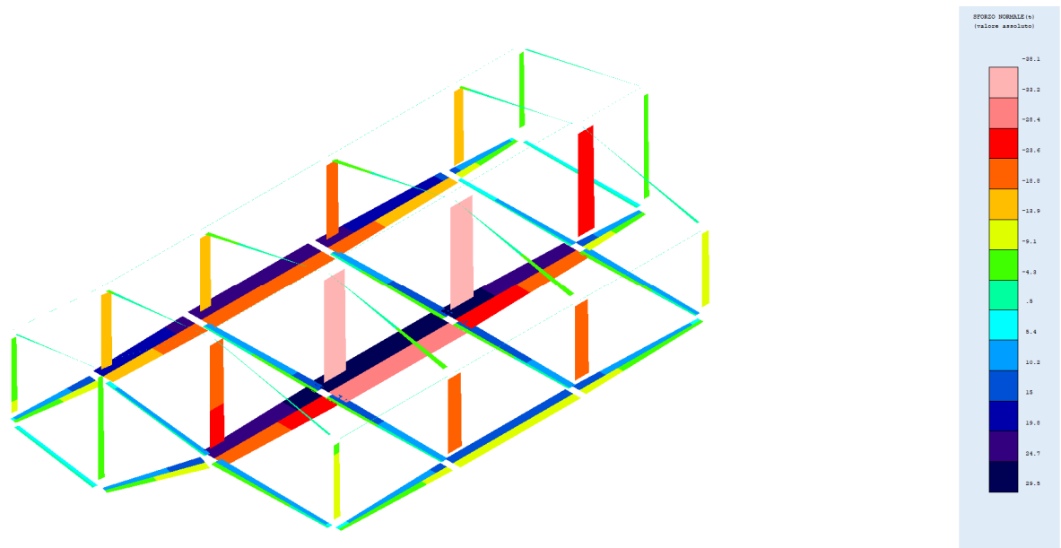
Fig. 59 –Sforzo normale
