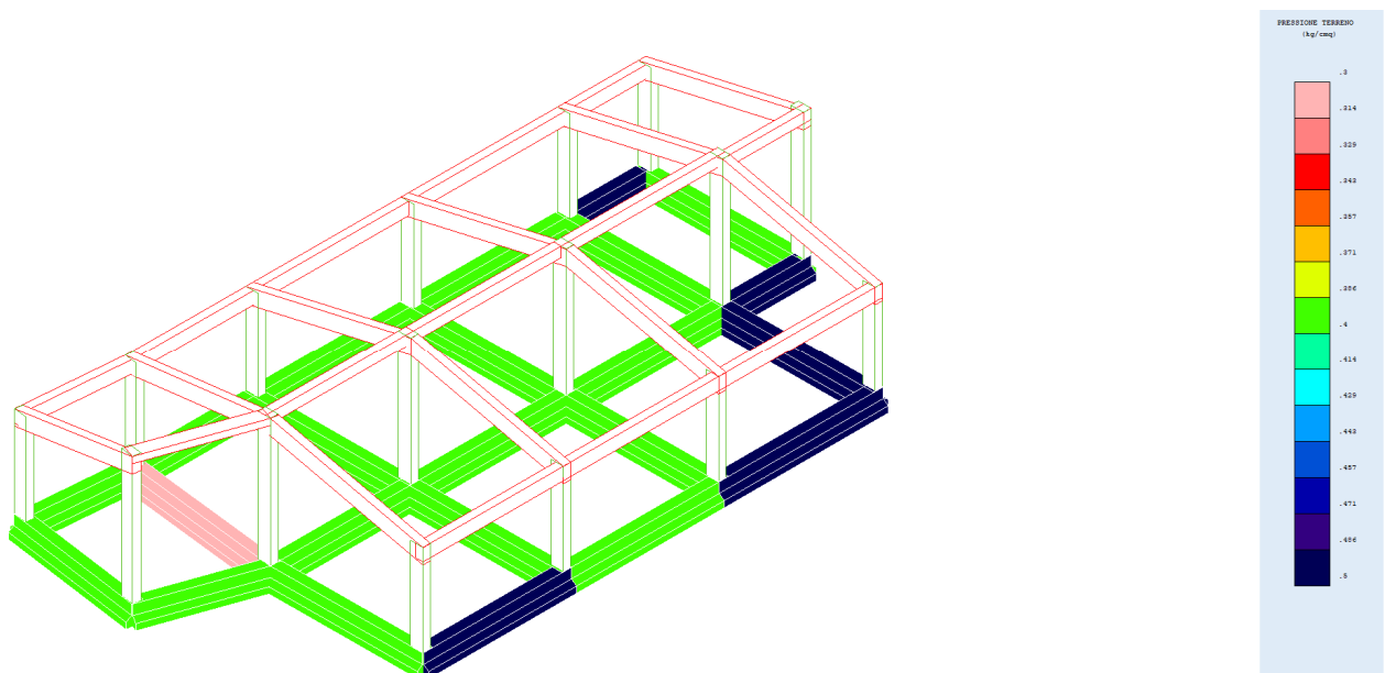
Fig. 57 – Pressione terreno
