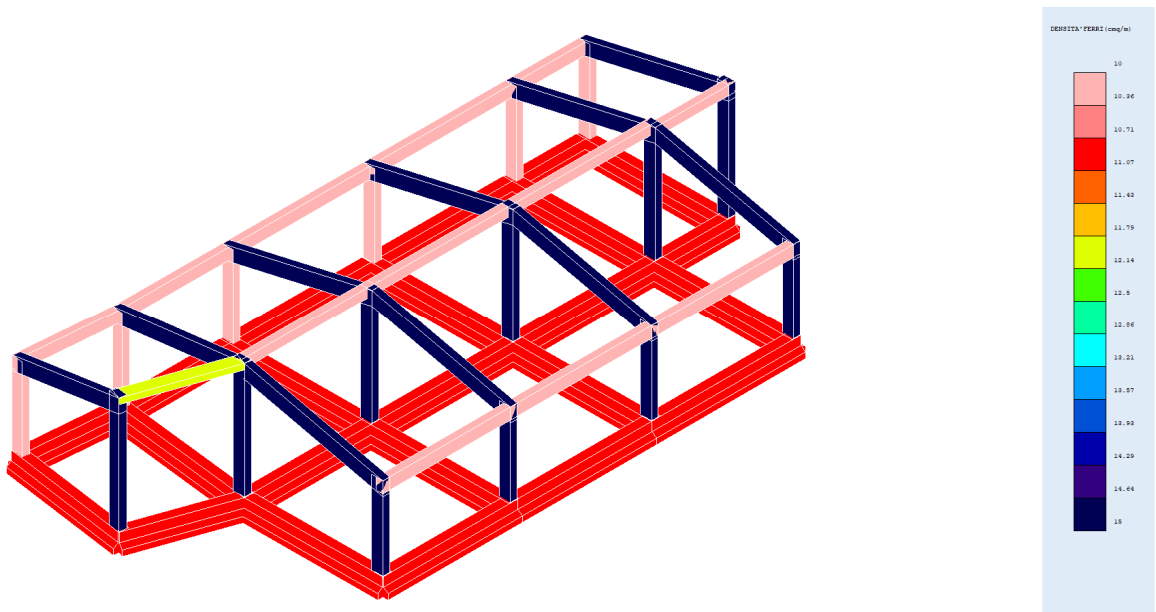
Fig. 55 – Densità ferri
