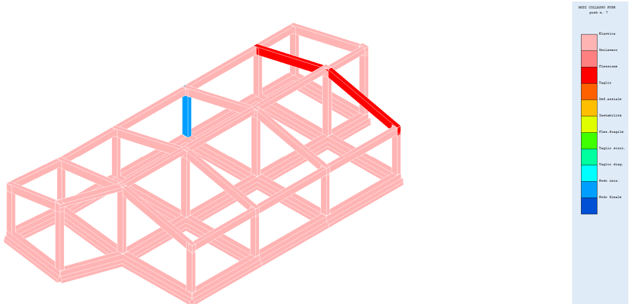
Fig. 44 – Modi collasso push 7
