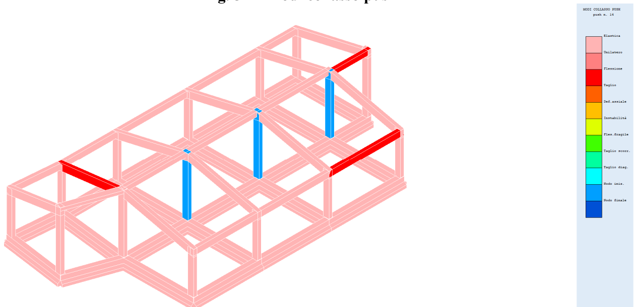
Fig. 51 – Modi collasso push 14
