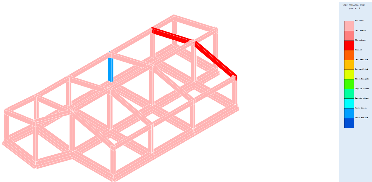
Fig. 40 – Modi collasso push 3
