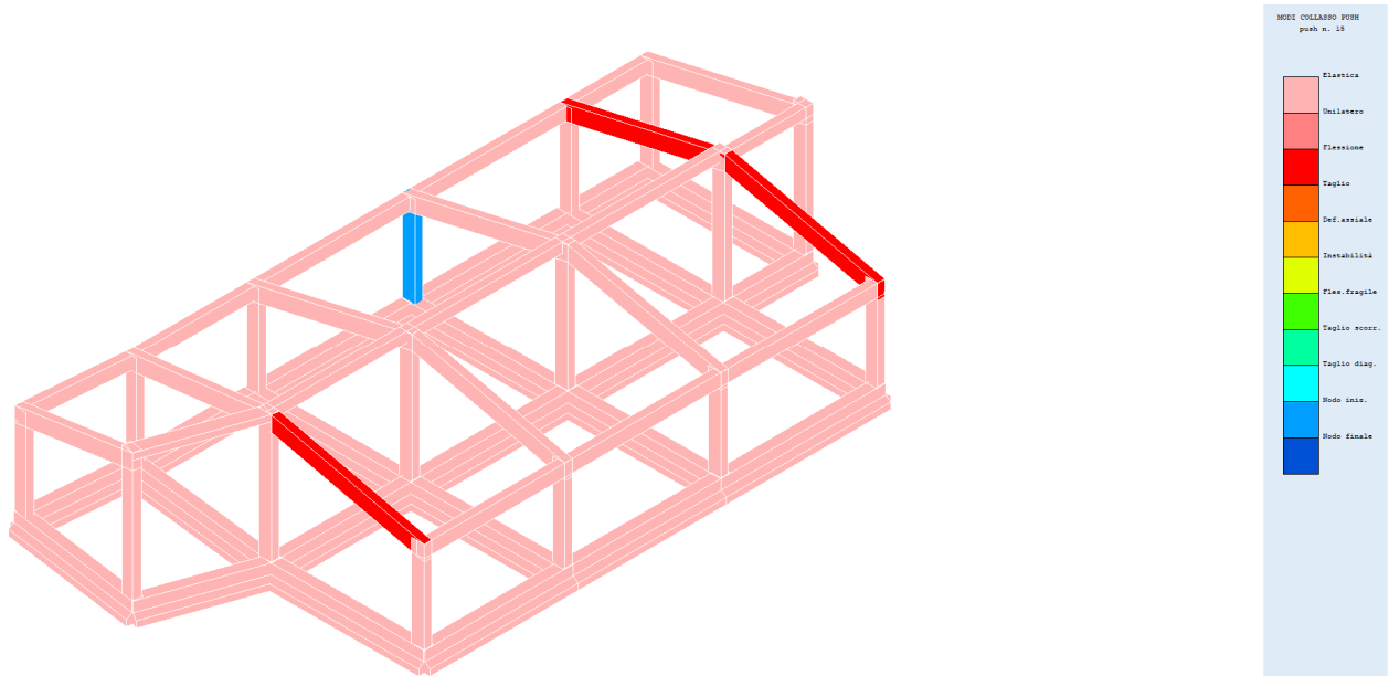
Fig. 52 – Modi collasso push 15
