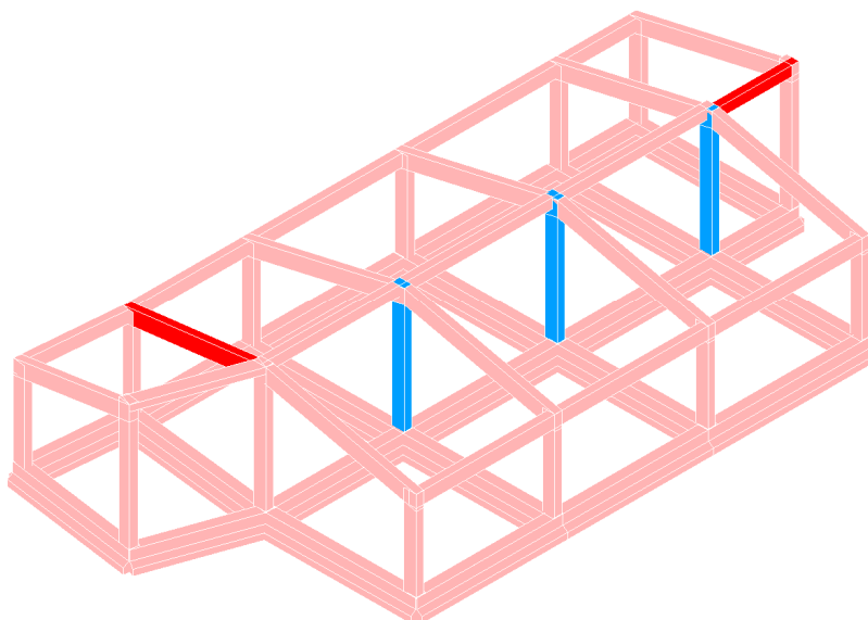
Fig. 47 – Modi collasso push 10
