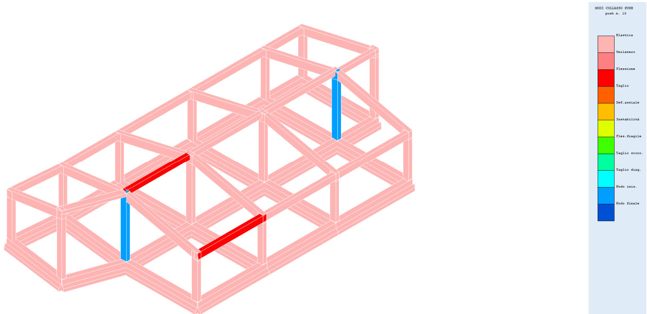
Fig. 50– Modi collasso push 13
