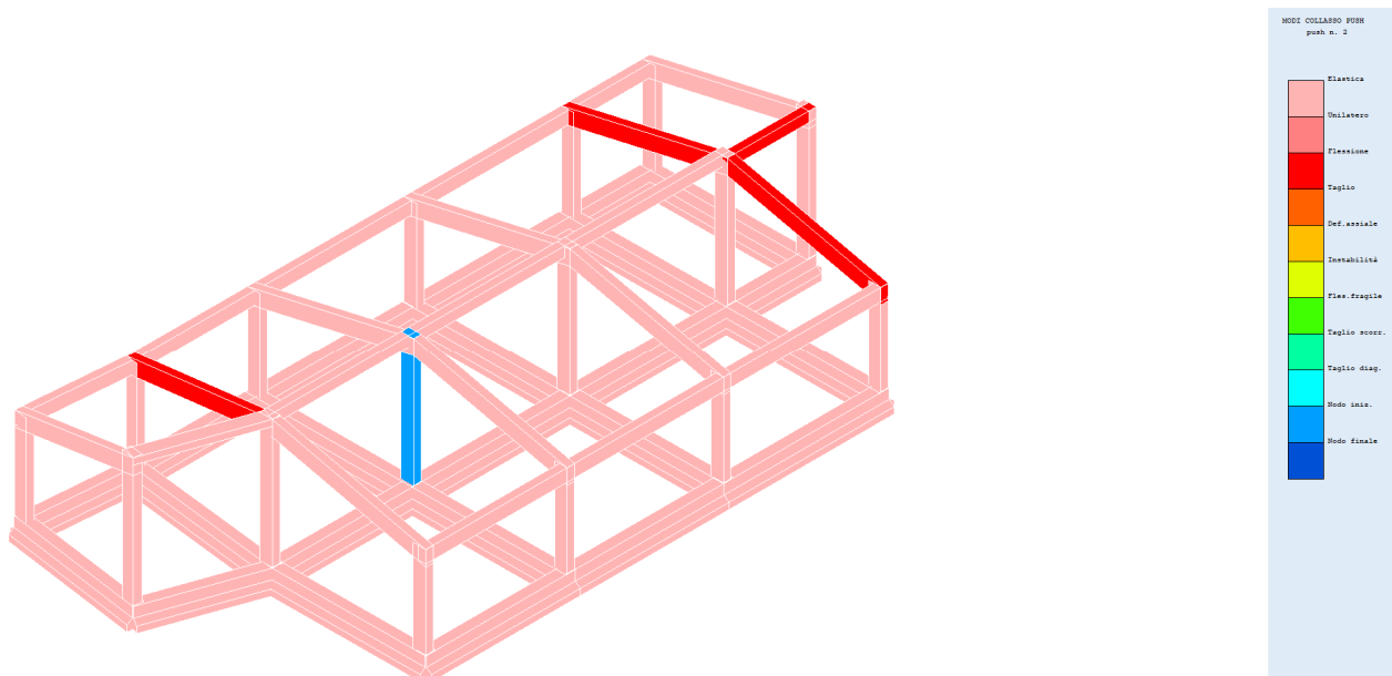
Fig. 39 – Modi collasso push 2
