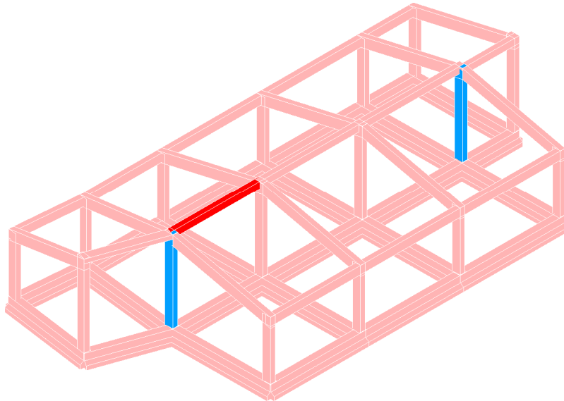
Fig. 46 – Modi collasso push 9
