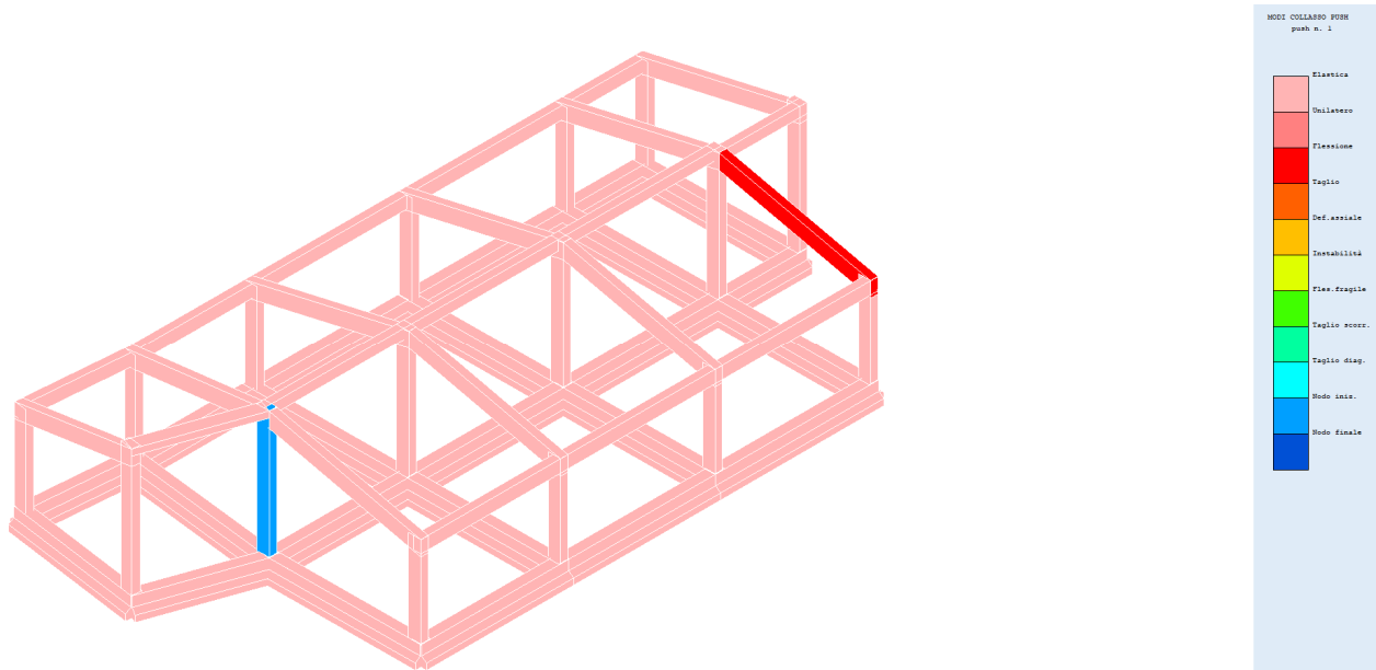
Fig. 38 – Modi collasso push 1
