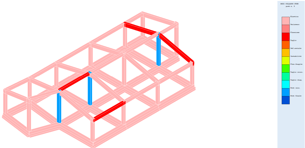
Fig. 42 – Modi collasso push 5
