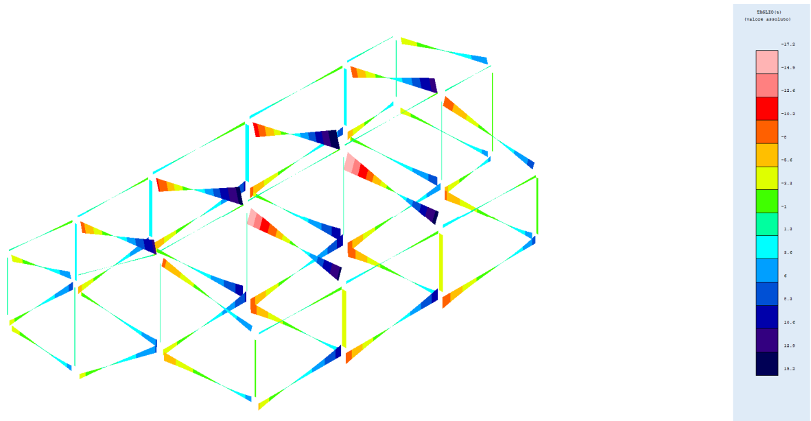
Fig. 60 – Taglio
