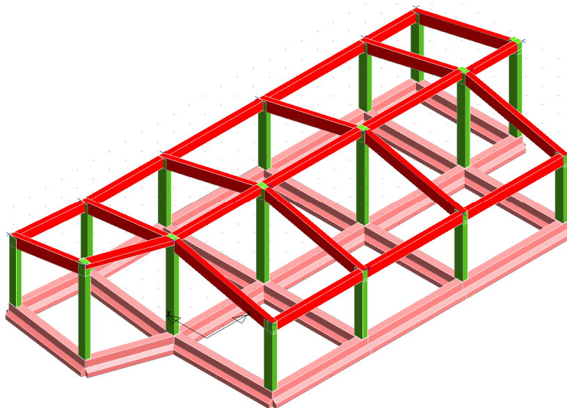
Fig. 2 – Schema struttura vista 3
