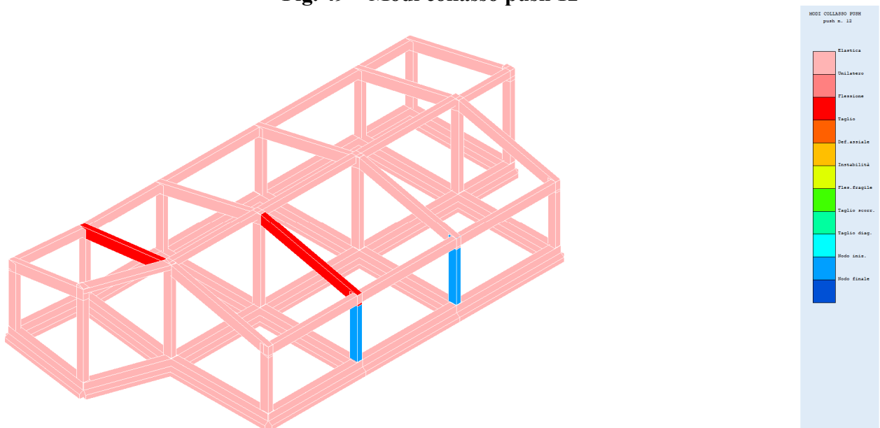
Fig. 49 – Modi collasso push 12
