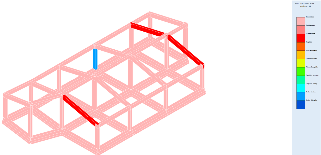
Fig. 48 – Modi collasso push 11
