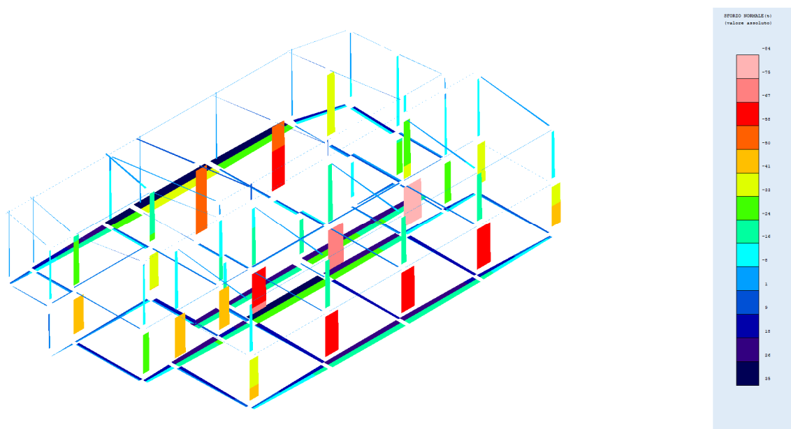
Fig. 75 – Sforzo Normale
