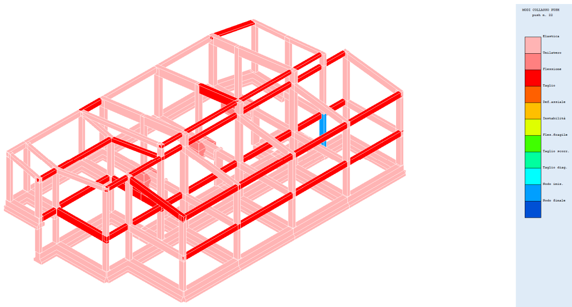
Fig. 59 – Modi collasso push 22
