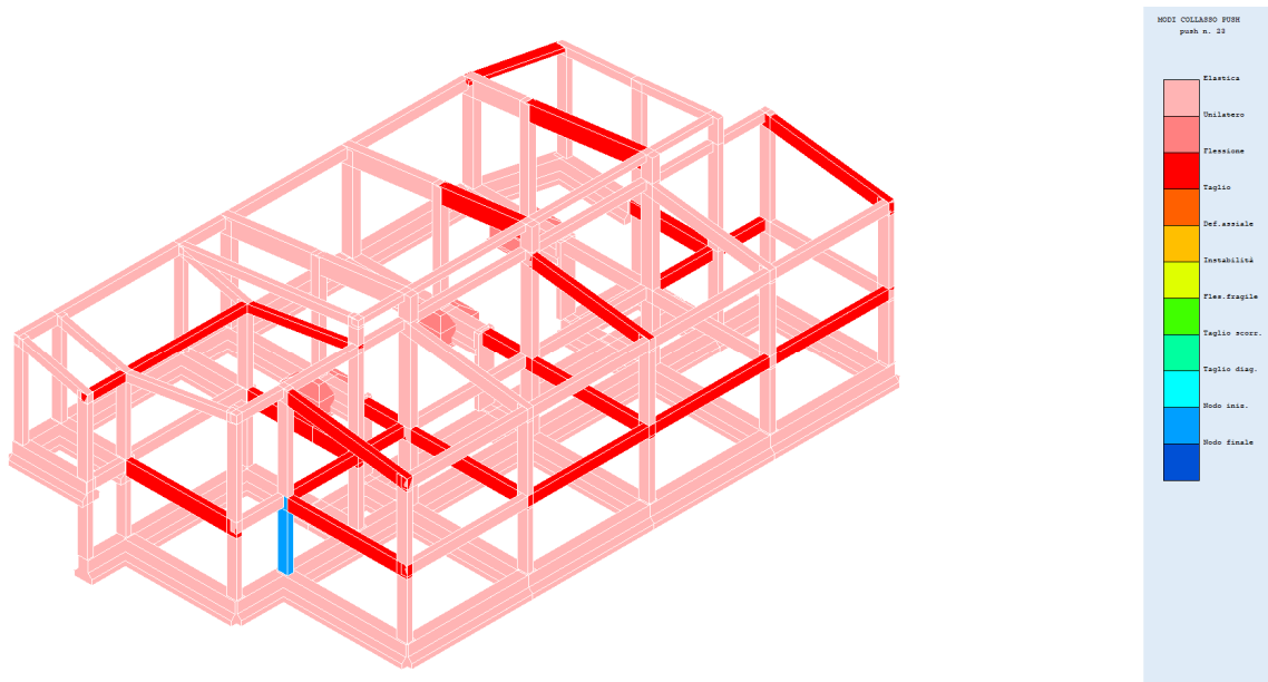
Fig. 60 – Modi collasso push 23
