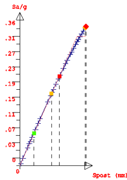
Fig. 8 – Push Over n° 4
