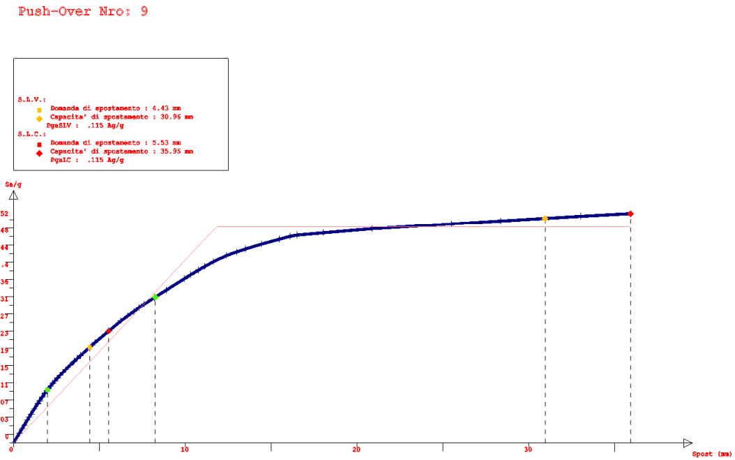
Fig. 13 – Push Over n° 9
