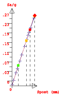
Fig. 36 – Push Over n°32
