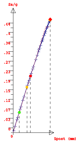
Fig. 12 – Push Over n° 8
