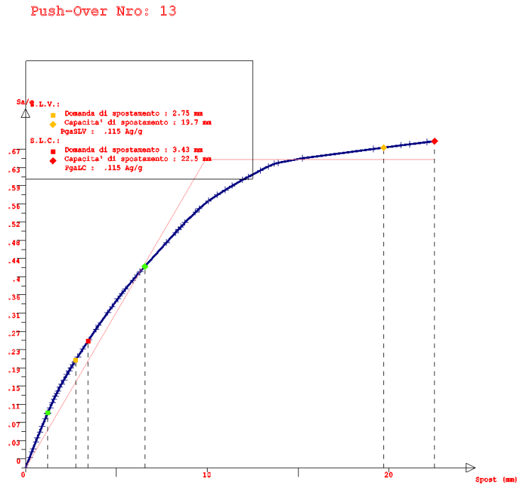
Fig. 17 – Push Over n° 13
