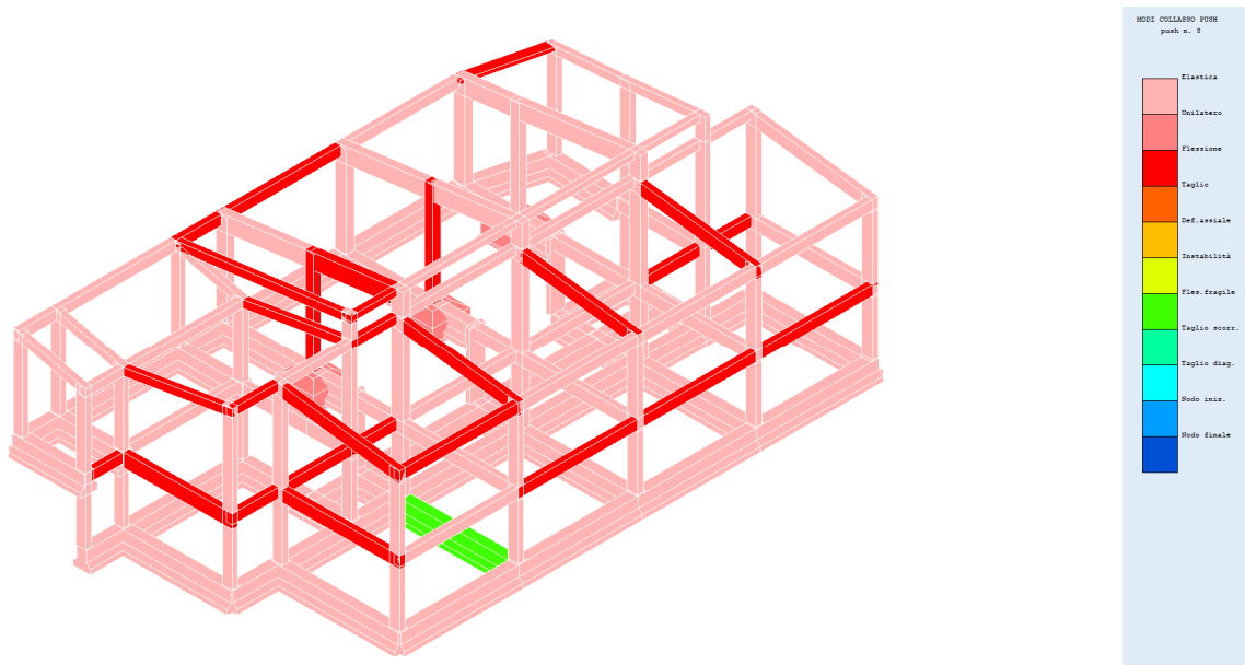
Fig. 45 – Modi collasso push 8
