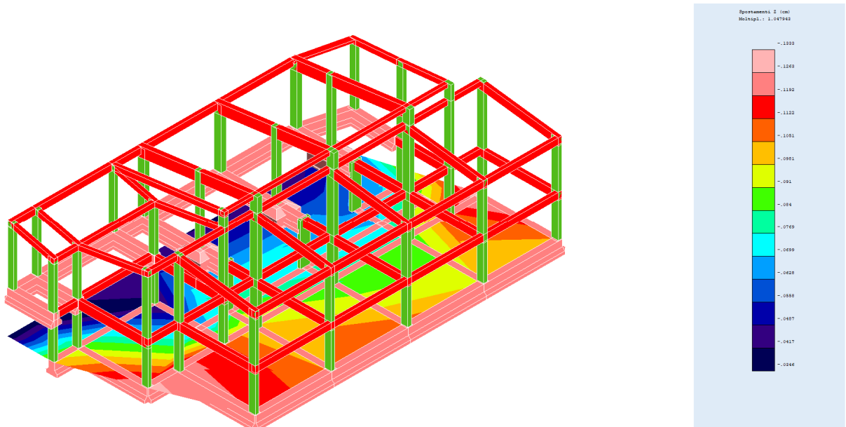
Fig. 79 – Fondazione - spostamenti Z
