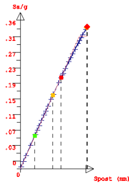
Fig. 24 – Push Over n°20
