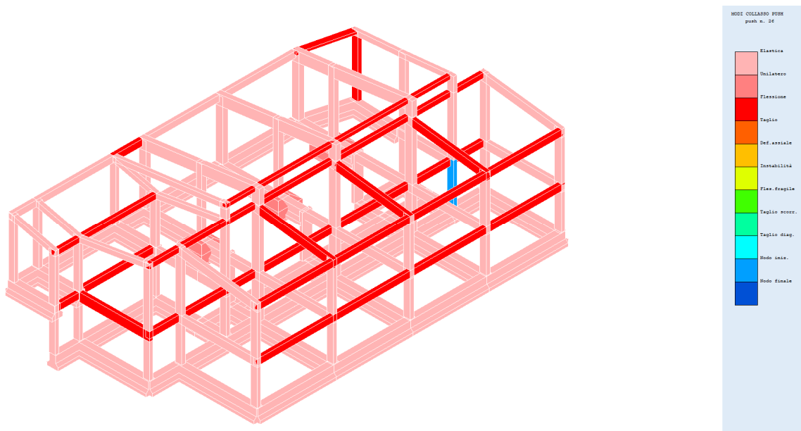
Fig. 63 – Modi collasso push 26
