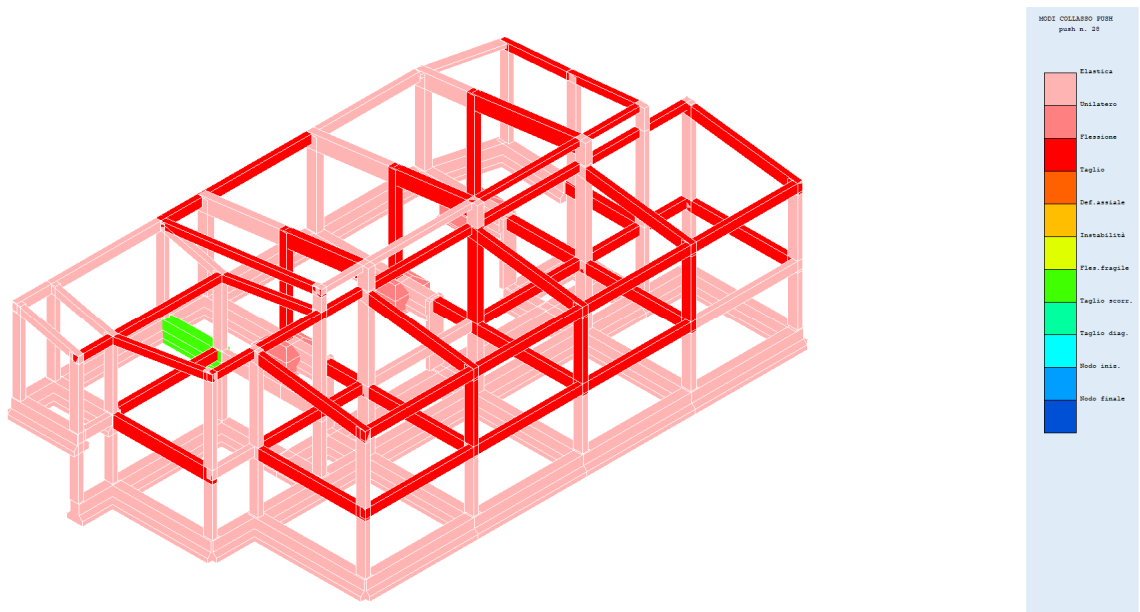
Fig. 65 – Modi collasso push 28
