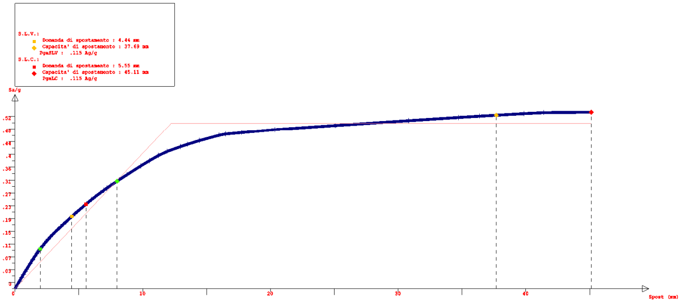
Fig. 30 – Push Over n°26
