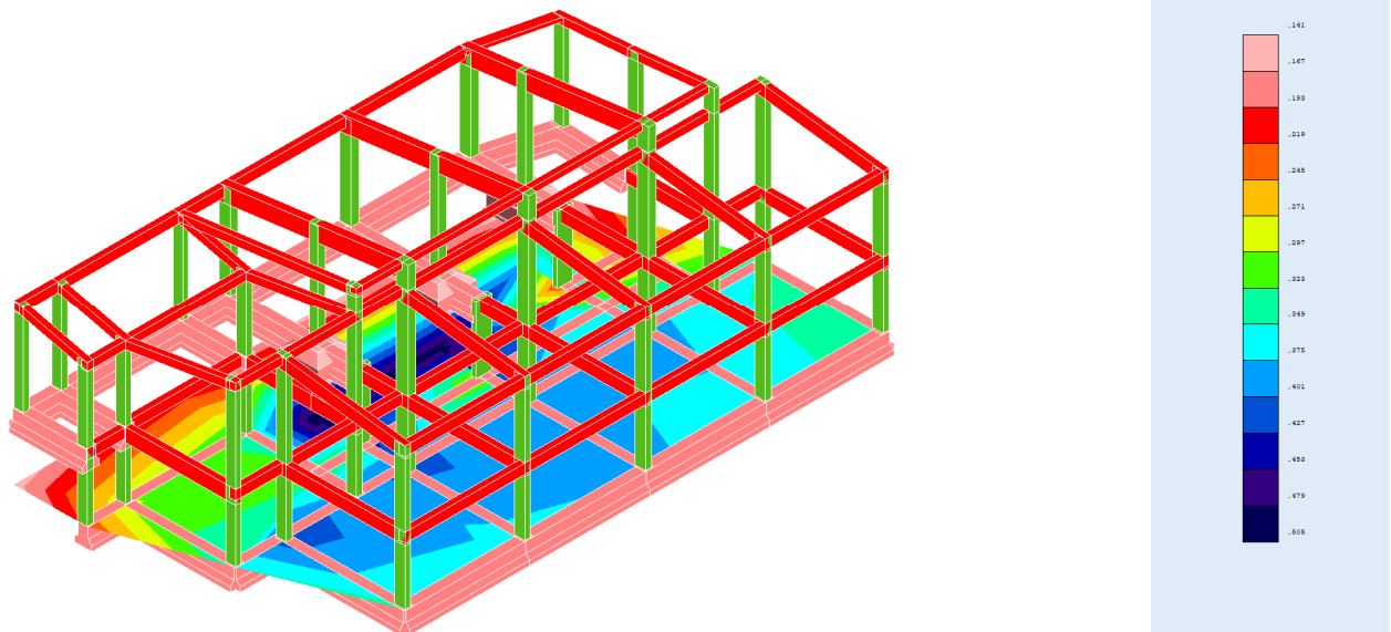
Fig. 77 – Cedimenti Edometrici
