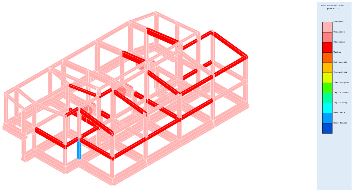
Fig. 64 – Modi collasso push 27
