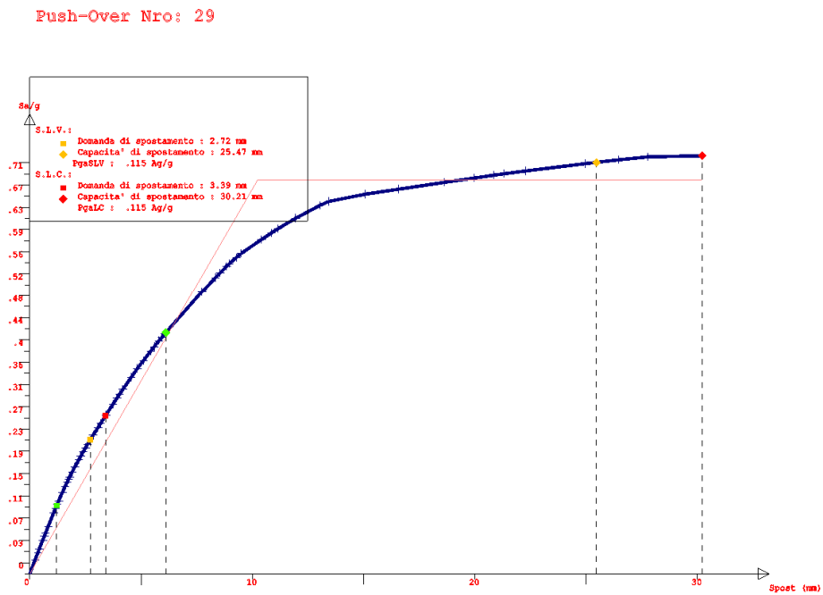
Fig. 33 – Push Over n°29
