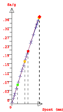
Fig. 20 – Push Over n° 16
