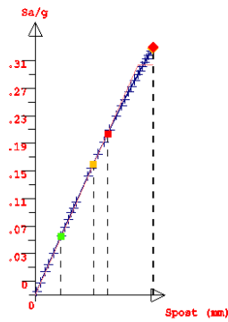
Fig. 16 – Push Over n° 12
