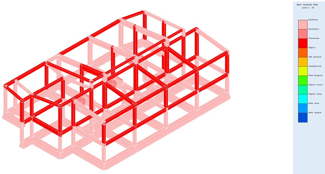
Fig. 62 – Modi collasso push 25
