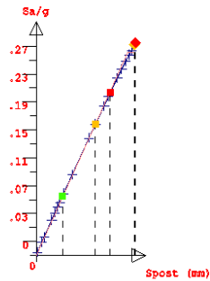
Fig. 32 – Push Over n°28
