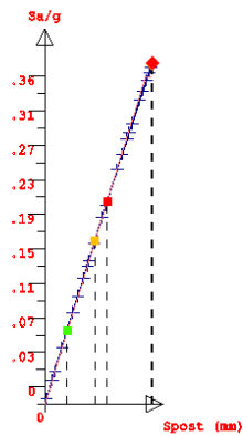
Fig. 28 – Push Over n°24
