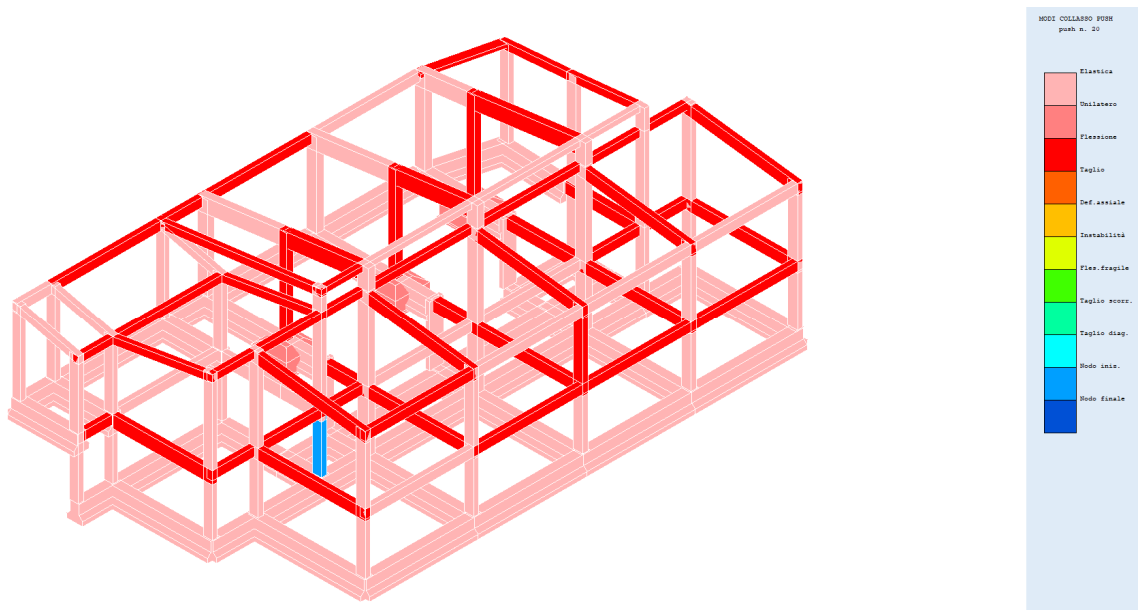
Fig. 57 – Modi collasso push 20
