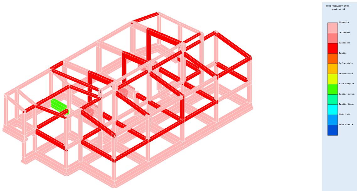
Fig. 49 – Modi collasso push 12
