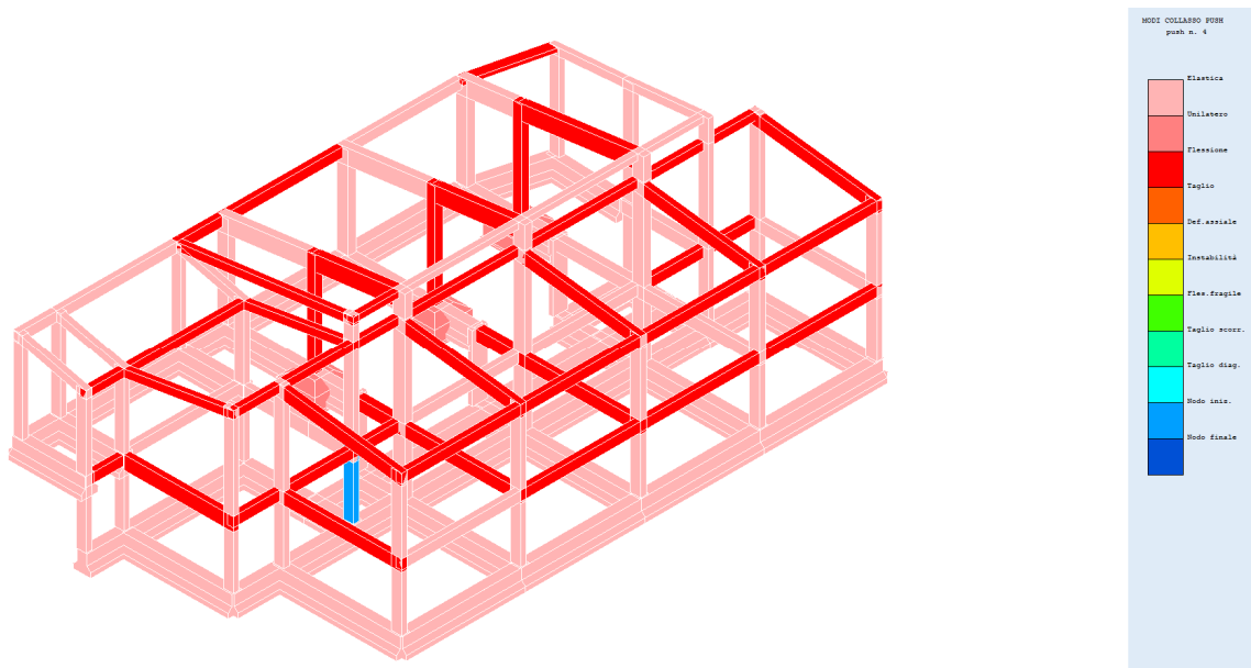
Fig. 41 – Modi collasso push 4
