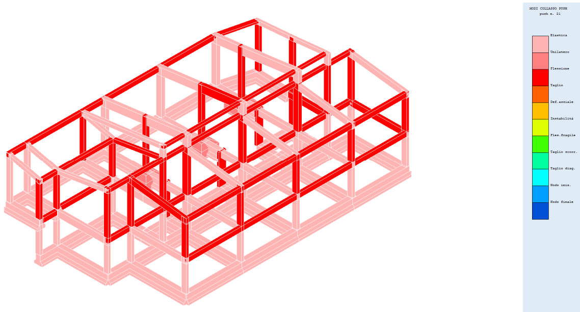
Fig. 58 – Modi collasso push 21
