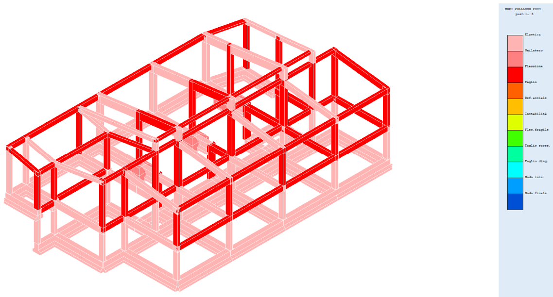
Fig. 42 – Modi collasso push 5
