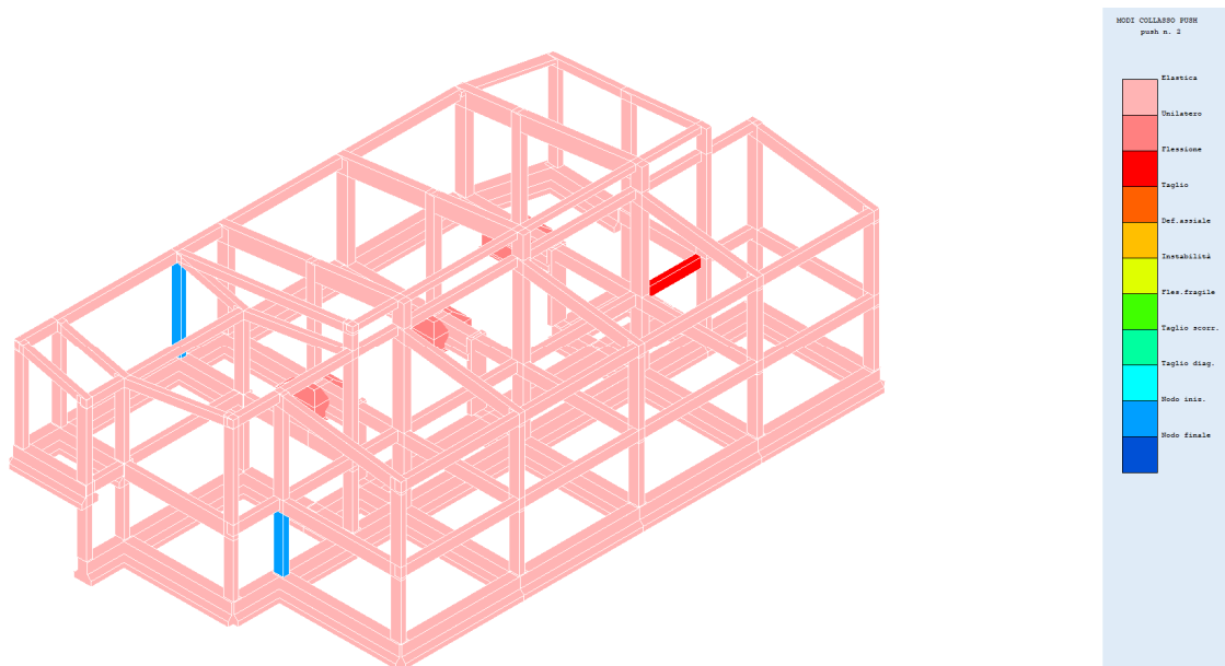
Fig. 39 – Modi collasso push 2
