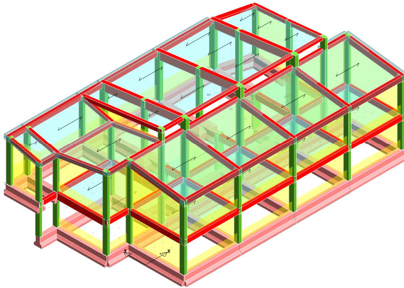
Fig. 4 – Schema struttura con carichi vista 3
