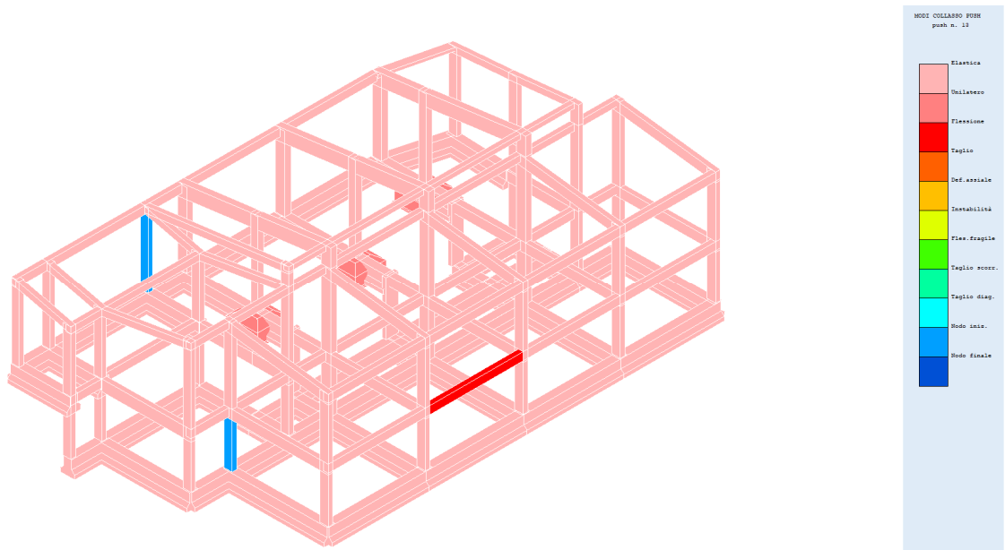
Fig. 50– Modi collasso push 13
