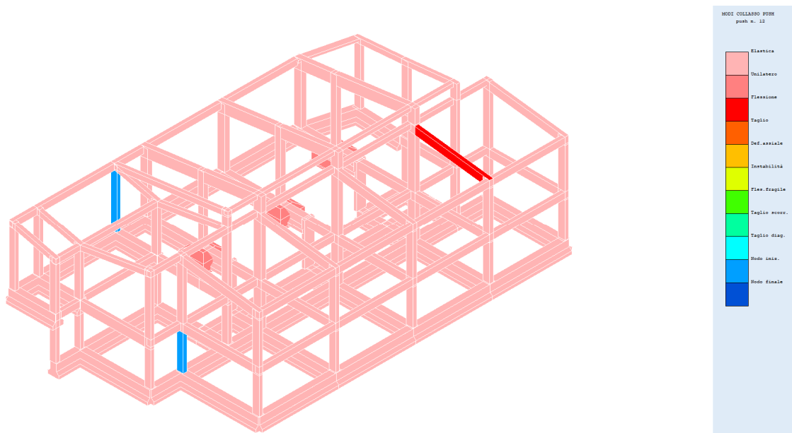
Fig. 49 – Modi collasso push 12
