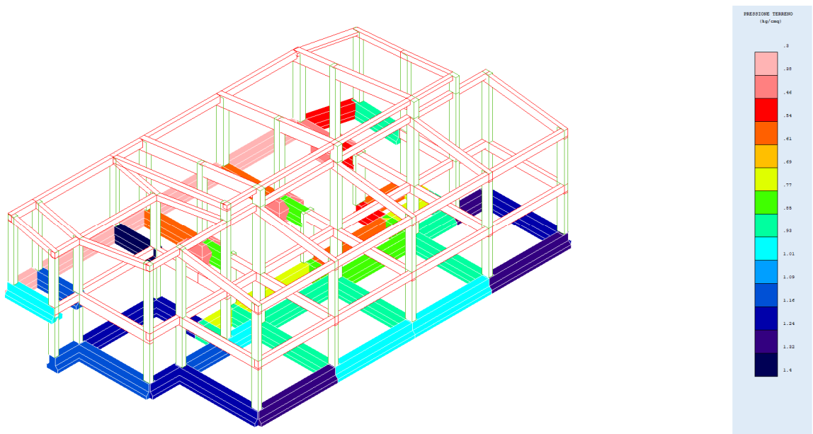
Fig. 57 – Pressione terreno
