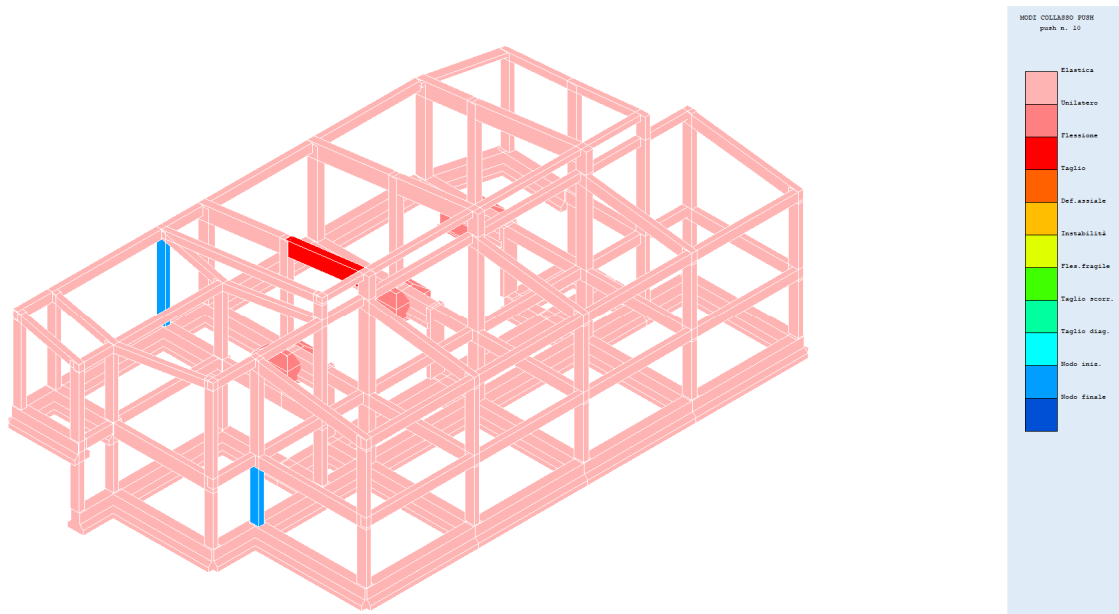
Fig. 48 – Modi collasso push 11
