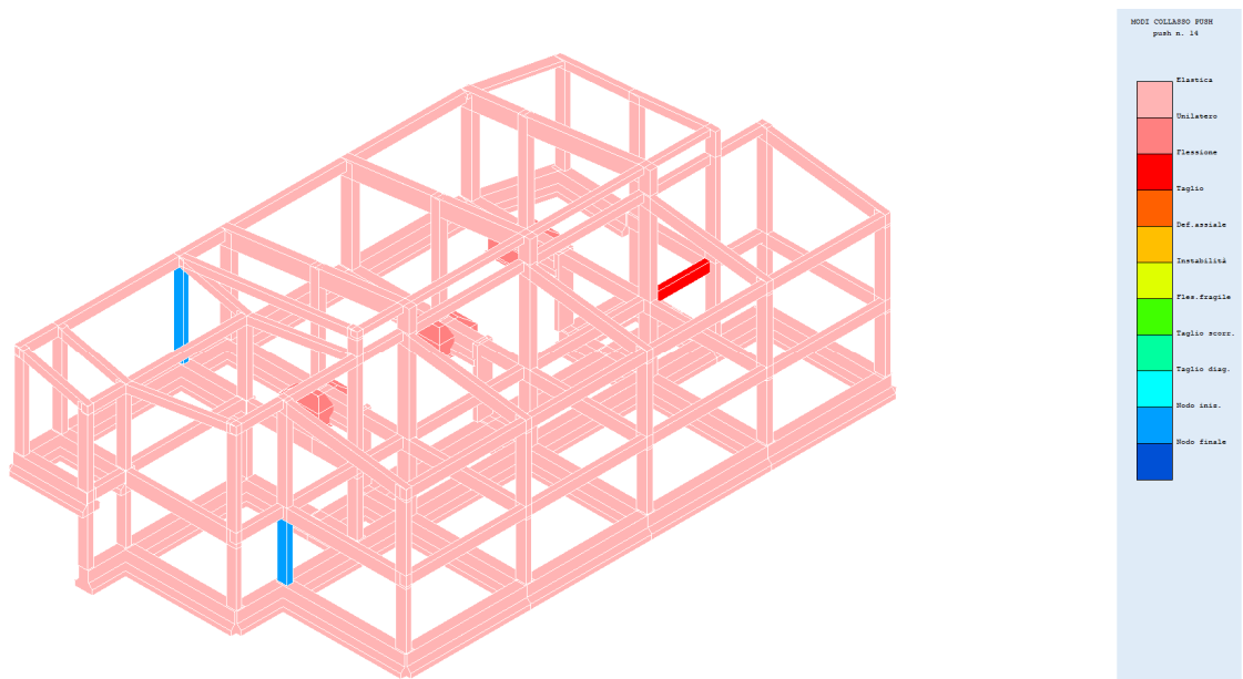
Fig. 51 – Modi collasso push 14
