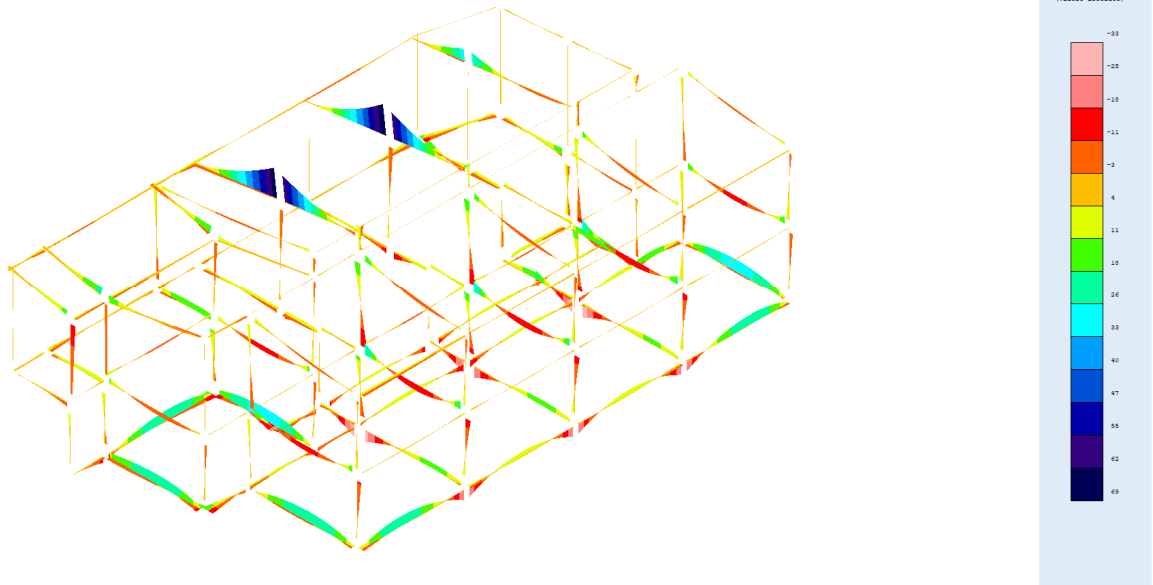
Fig. 58 –Momento involuppo
