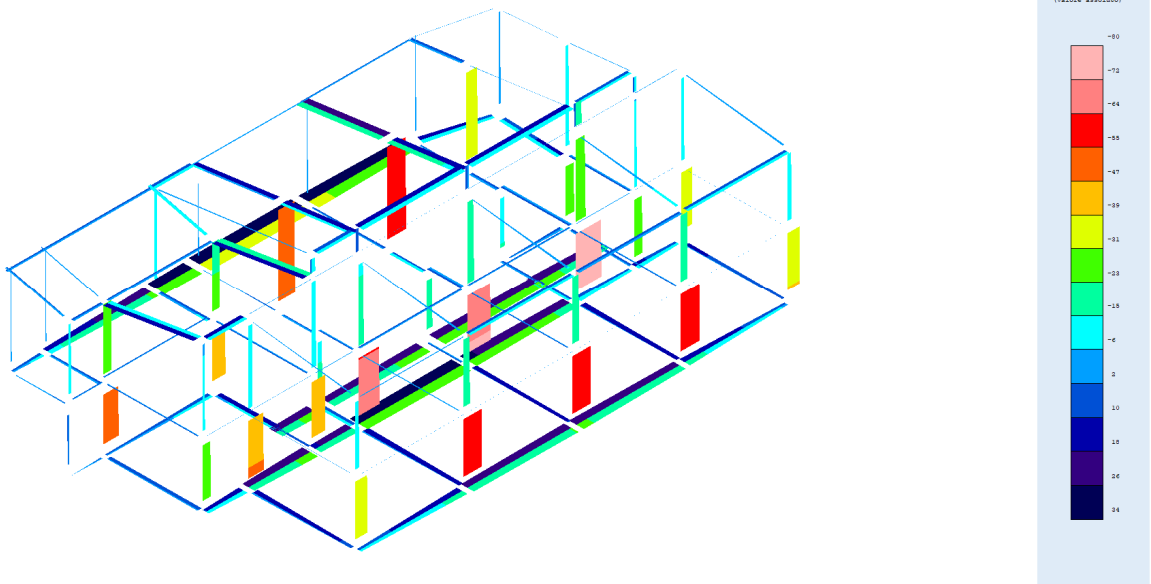
Fig. 59 –Sforzo normale
