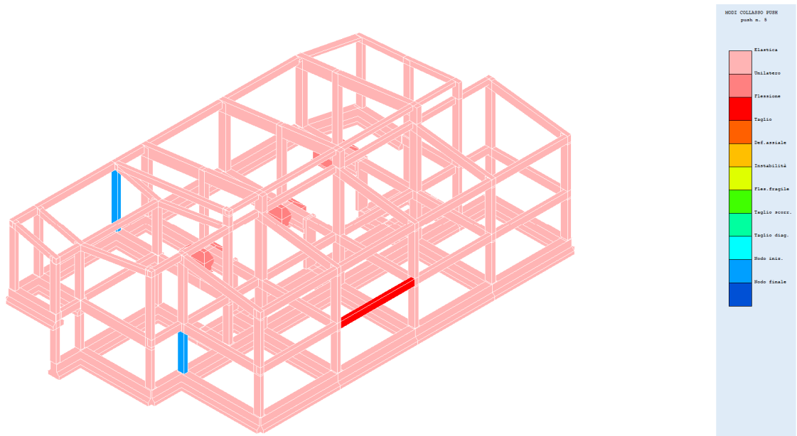
Fig. 42 – Modi collasso push 5
