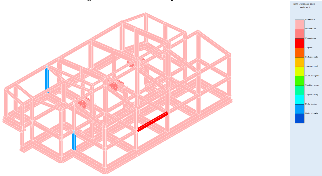
Fig. 38 – Modi collasso push 1
