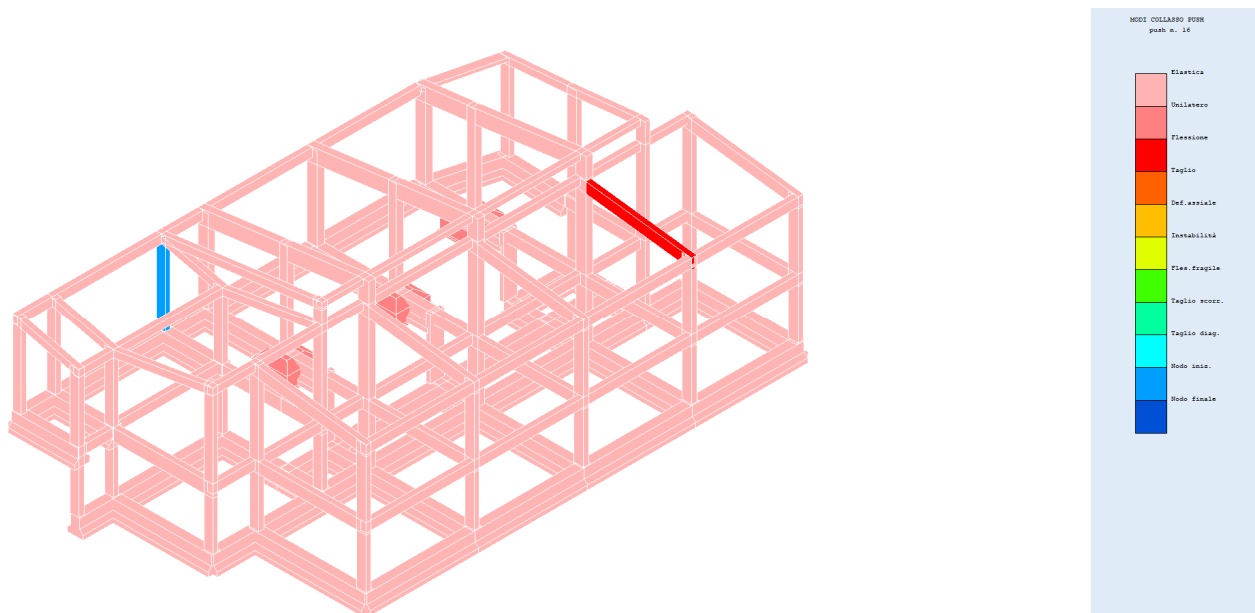
Fig. 53 – Modi collasso push 16
