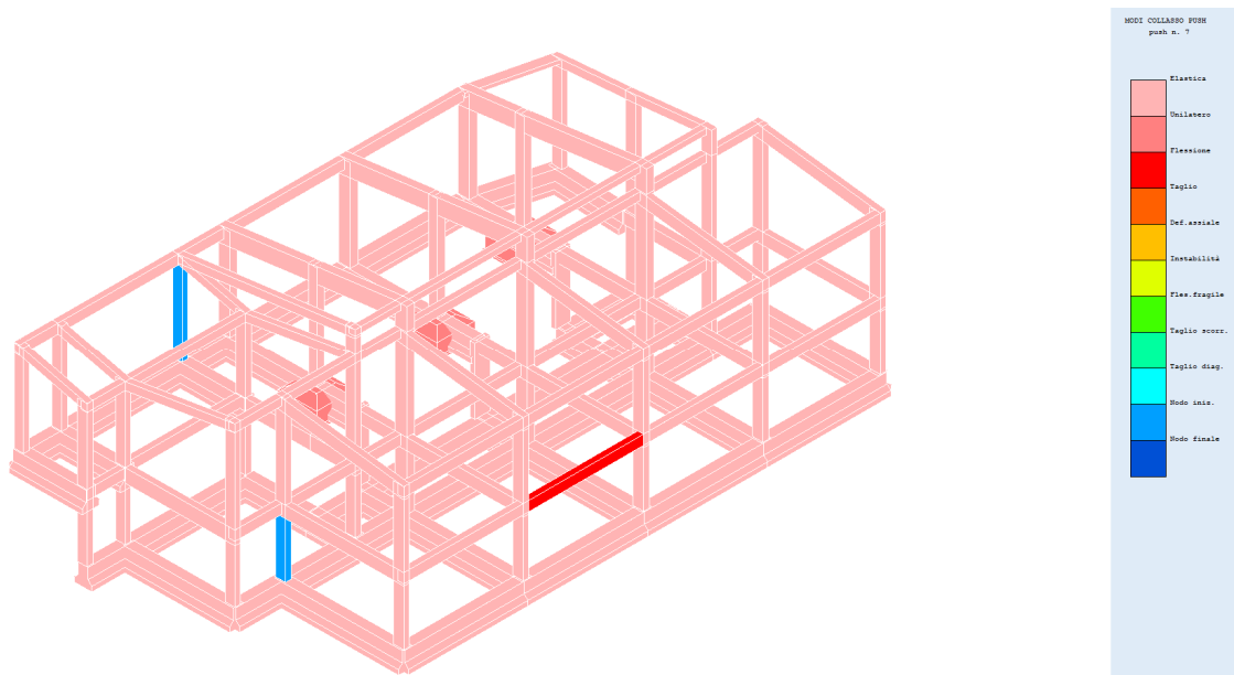
Fig. 44 – Modi collasso push 7
