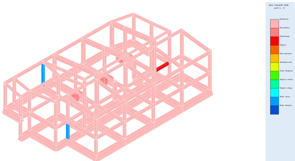
Fig. 47 – Modi collasso push 10
