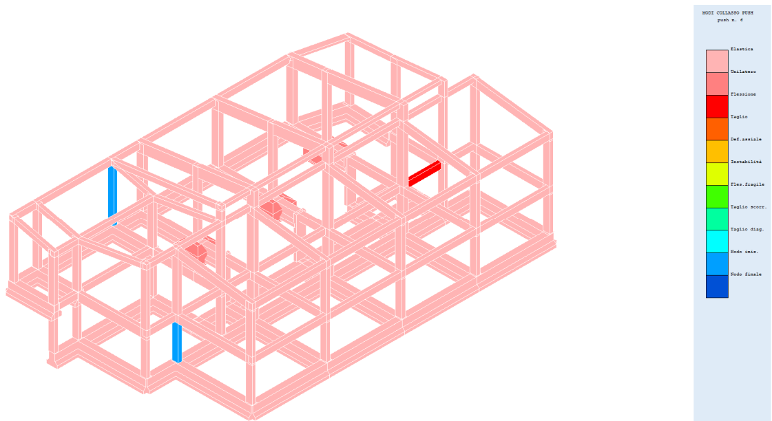
Fig. 43 – Modi collasso push 6
