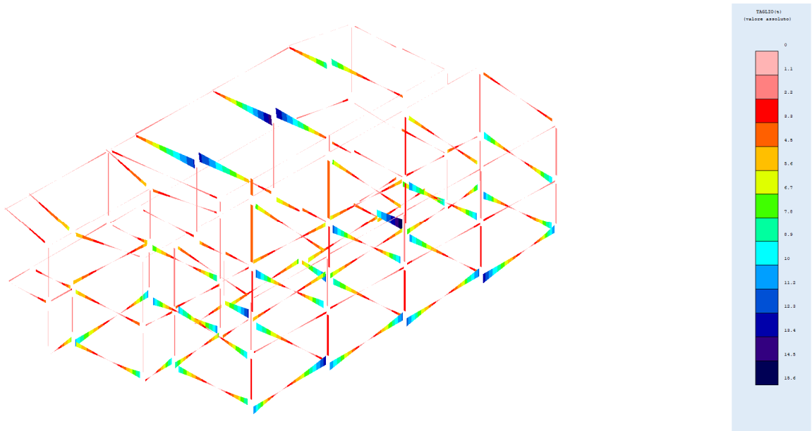
Fig. 60 – Taglio
