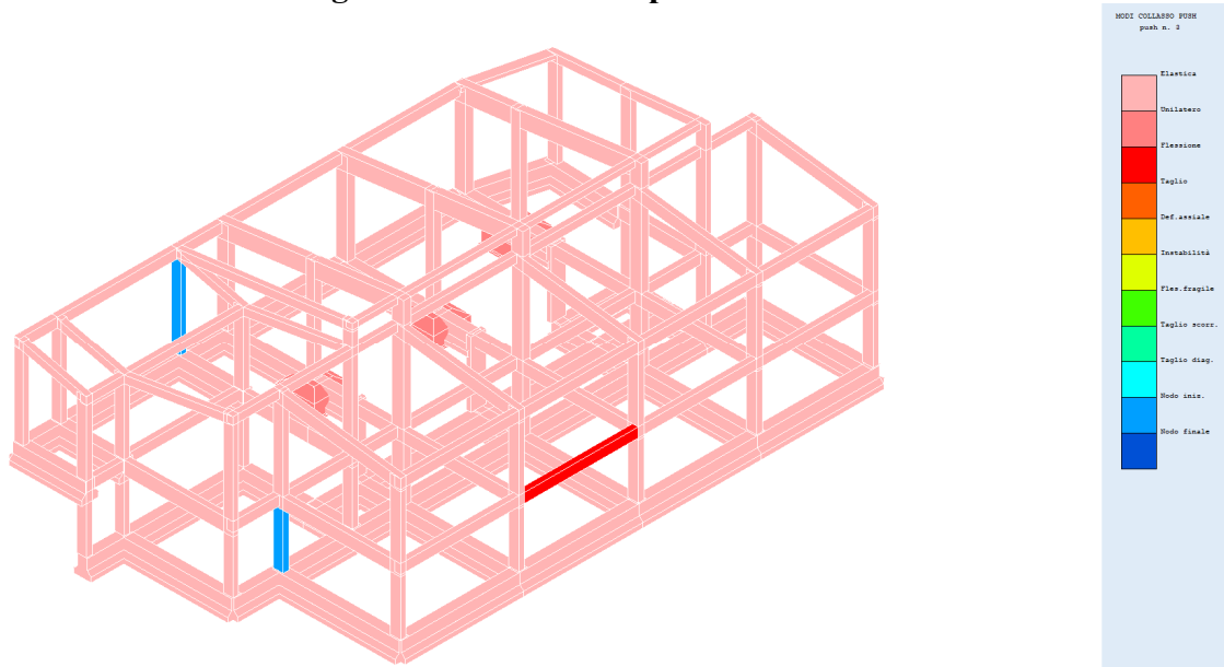
Fig. 40 – Modi collasso push 3
