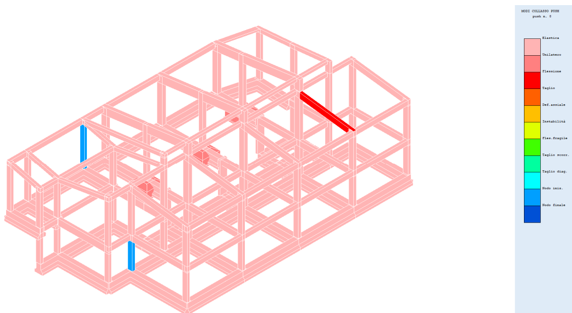
Fig. 45 – Modi collasso push 8
