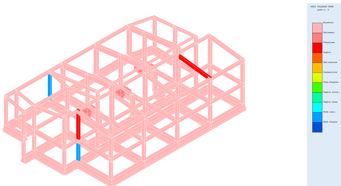
Fig. 41 – Modi collasso push 4
